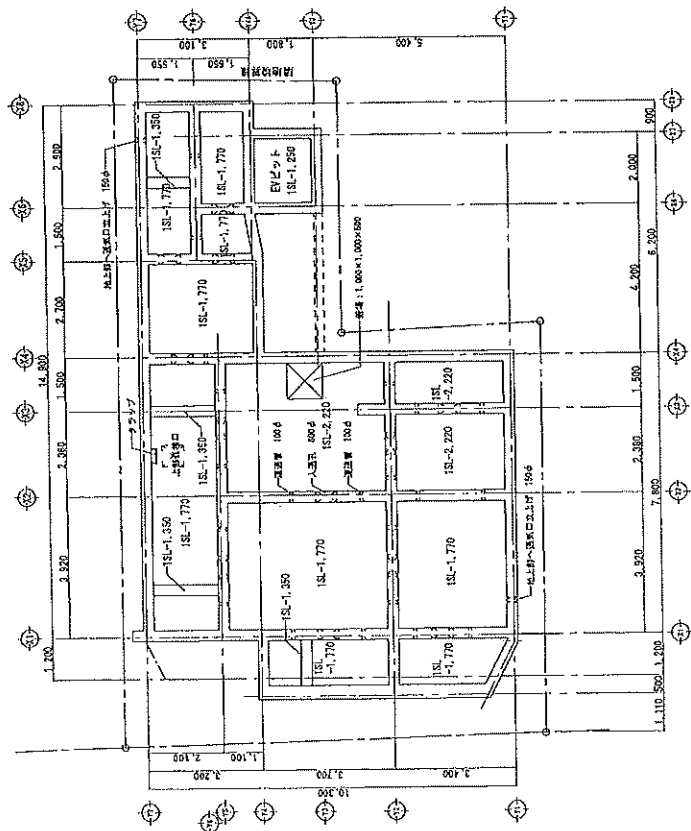
1階平面図 1/100
