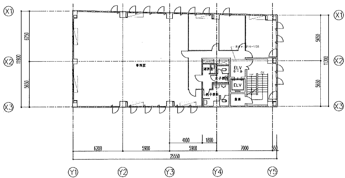
4階平面図
