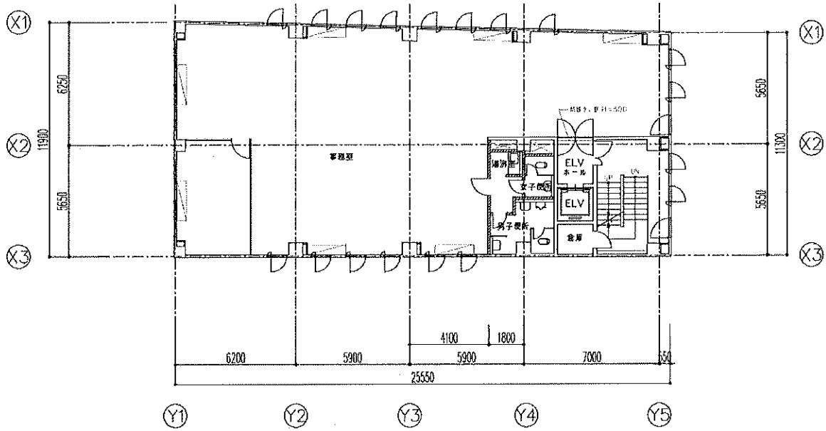
3階平面図
