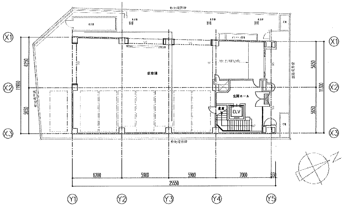
1階平面図
