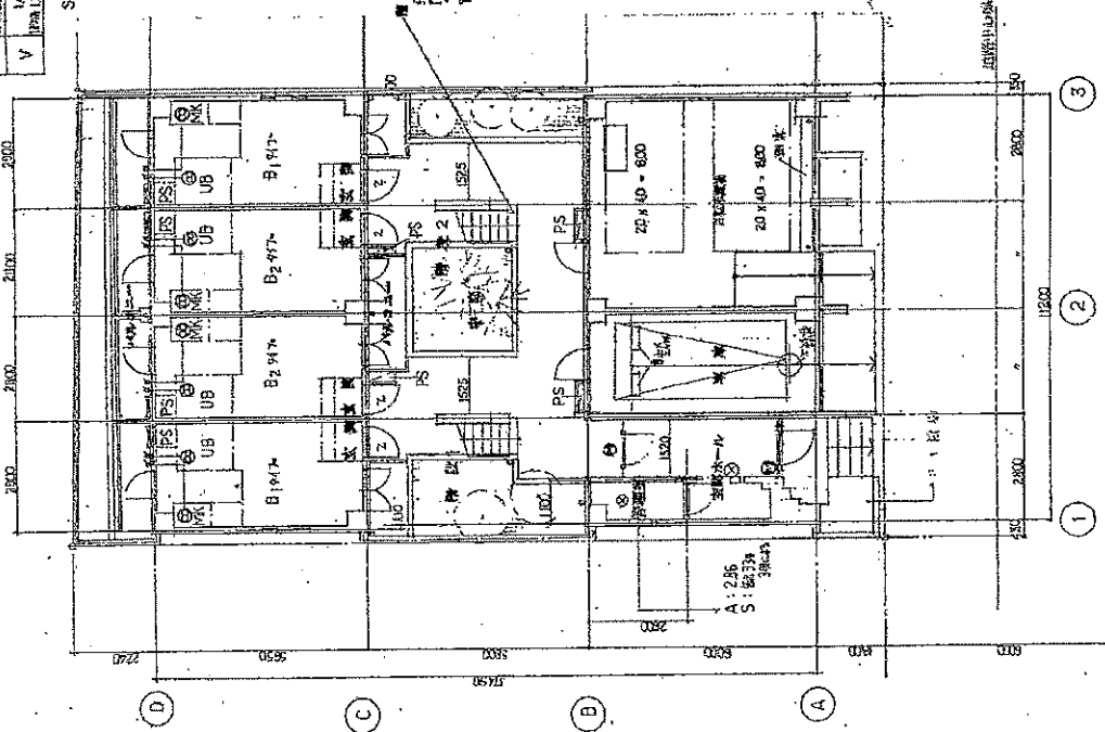
1階平面図
